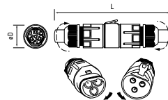
PCC-I3-FD 3x1.5 16A IP68
