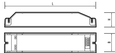
PEPP40-1.0H U IP20 (Габаритные размеры)
