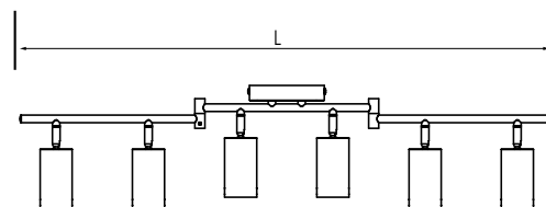
Рис.4 Светильник PCL 0606
